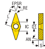
VBMT-MF2
