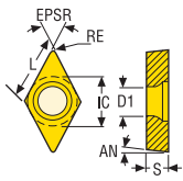
DCMW
